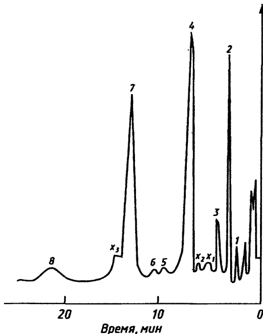
1 — бензол; 2 — акрилонитрил; 3 — толуол; 4 — этилбензол; 5 — м-ксилол; 6 — изопропилбензол; 7 — стирол; 8 — α-метилстирол; x_1 , x_2 , x_3 — неидентифицированные компоненты
