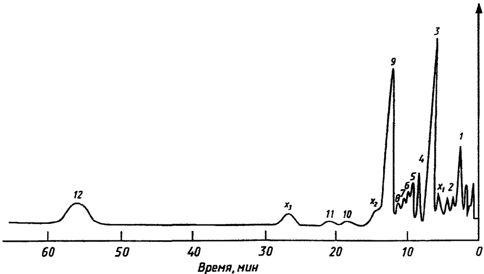
1 — бензол; 2 — толуол; 3 — этилбензол; 4 — n -ксилол; 5 — m -ксилол; 6 — изопропилбензол; 7 — o -ксилол; 8 — n -пропилбензол; n -метилэтилбензол; m -этилтолуол; 9 — стирол; 10 — фенилацетилен; 11 — α -метилстирол; 12 — бензальдегид; x 1 , x 2 , x 3 — неидентифицированные компоненты
