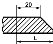
Рисунок 4 — Присоединительный конец под приварку
