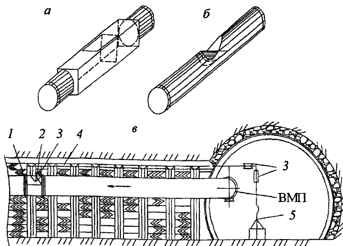
Рис. 1. Устройство для разгазирования тупиковых горных выработок: а, б - схемы устройства; в - схема установки; 1 - патрубкок; 2 - клапан; 3 - ролики; 4 - трос; 5 - ручная (электрическая) лебедка
