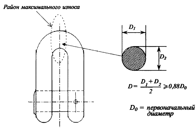
Рис. 3 Места замеров звена цепи и максимально допустимый износ
