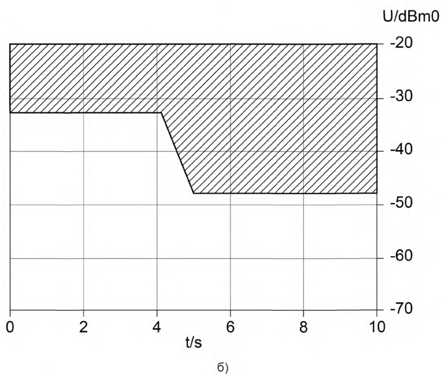
Рисунок И.1 — Зависимость степени подавления эхосигналов L и уровня эхосигналов U от времени
