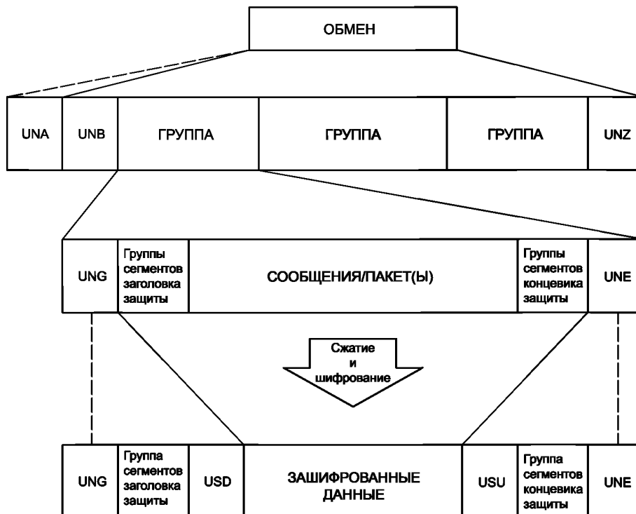
Рисунок 2 — Схематическое представление структуры обмена, содержащего одну группу, информационное наполнение которой (тело группы и ассоциируемые с ним группы сегментов заголовка и конца заголовка защиты) было зашифровано
