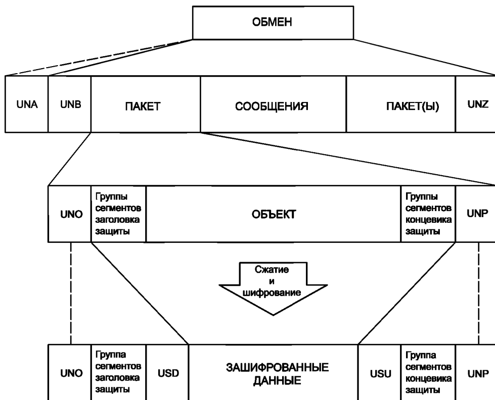
Рисунок 4 — Схематическое представление структуры обмена с одним пакетом, информационное наполнение которого (объект и ассоциируемые с ним группы сегментов заголовка и концевого заголовка защиты) были зашифрованы
