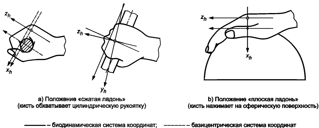
Рисунок 2 — Базицентрическая и биодинамическая системы координат кисти руки
