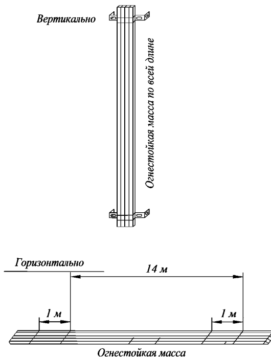
Рис. 16.8.4.3.2-1 Защита кабельной трассы огнестойкой массой
