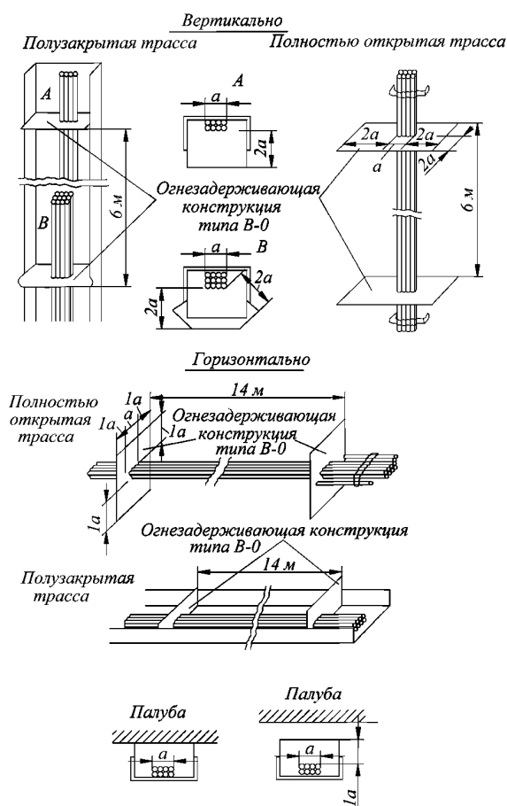
Рис. 16.8.4.3.2-2 Защита кабельных трасс огнезадерживающими конструкциями типа В-О
