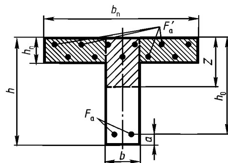
Рис. 7.3.40-2. К расчету статических моментов S_{\bar{0}} и S_0
