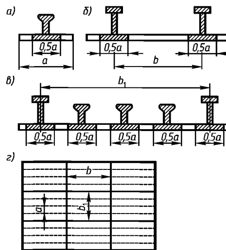
Рис. 3.3.2.1. Определение ширины присоединенного пояска продольных ребер
