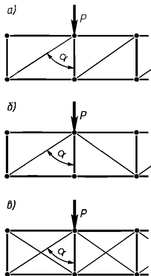
Рис. 2.2.55. Варианты ферм
