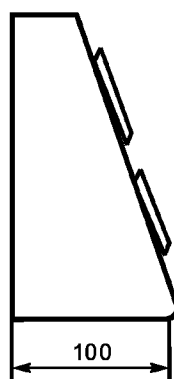
Рисунок F.1 — Пример управления XL устройства в кабине лифта (вид сбоку)
