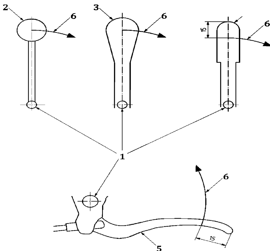
1 — точка поворота рычага; 2 — рычаг со сферической головкой; 3 — конусообразный рычаг; 4 — параллельный рычаг; 5 — рычаг типа велосипедного тормоза; 6 — траектория точки приложения силы
