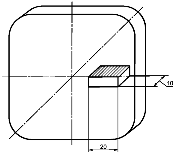
Рисунок 1 — Образец от прутка или заготовки с диаметром или длиной стороны свыше 40 мм
