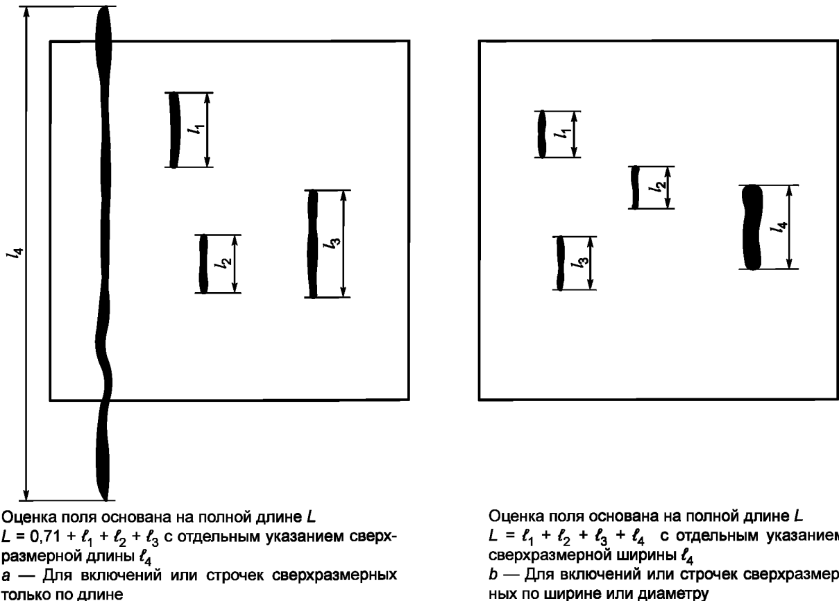
Рисунок В.2 — Оценка поля со сверхразмерными включениями или строчками
