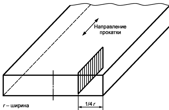
Рисунок 4 — Образец от листа толщиной не более 25 мм
