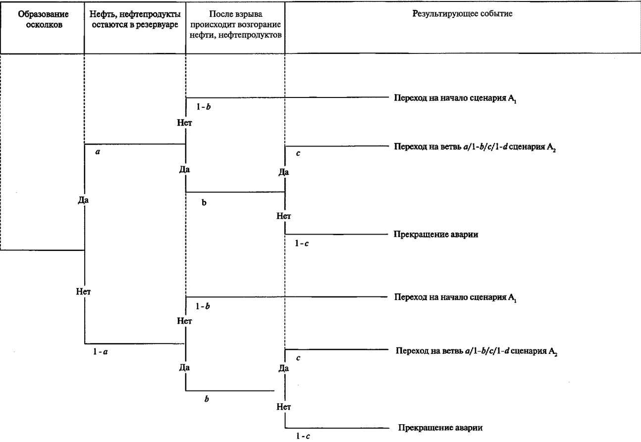
Рис. 1-3. Дерево событий при взрыве внутри наземного резервуара
