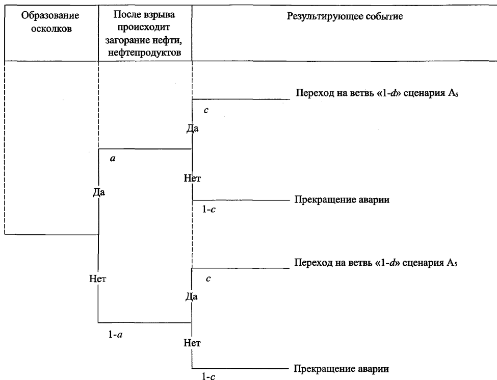
Рис. 1-6. Дерево событий при взрыве внутри подземного резервуара (типа ЖБР)
