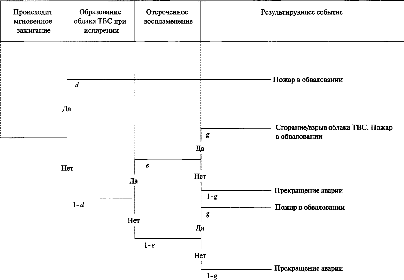
Рис. 1-4. Дерево событий разрушения/перелива подземного резервуара
