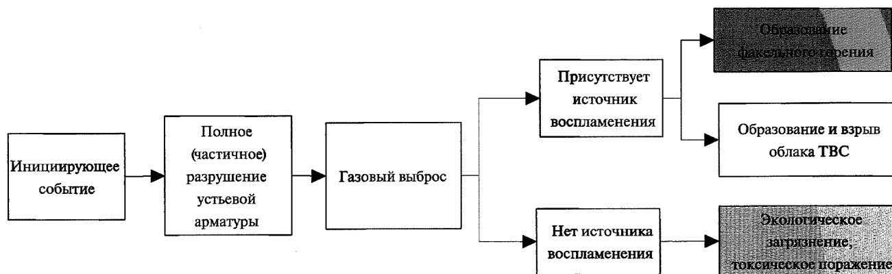
Рис. 1-11. Скважины газовые
