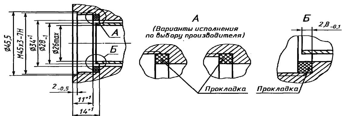
Рисунок Б.4 — Резьбовое соединение с внутренней резьбой для систем с двумя каналами подачи воздуха PIV
