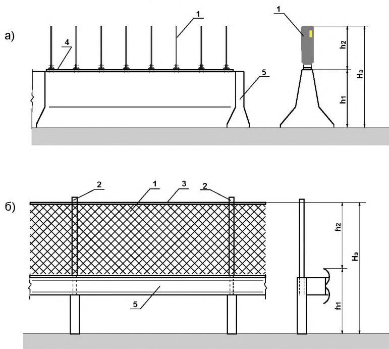
Рисунок 1 – Схема задерживания экраном светового потока
