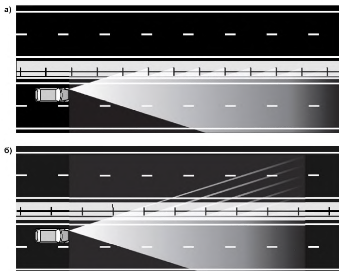
Рисунок 1 – Схема задерживания экраном светового потока
