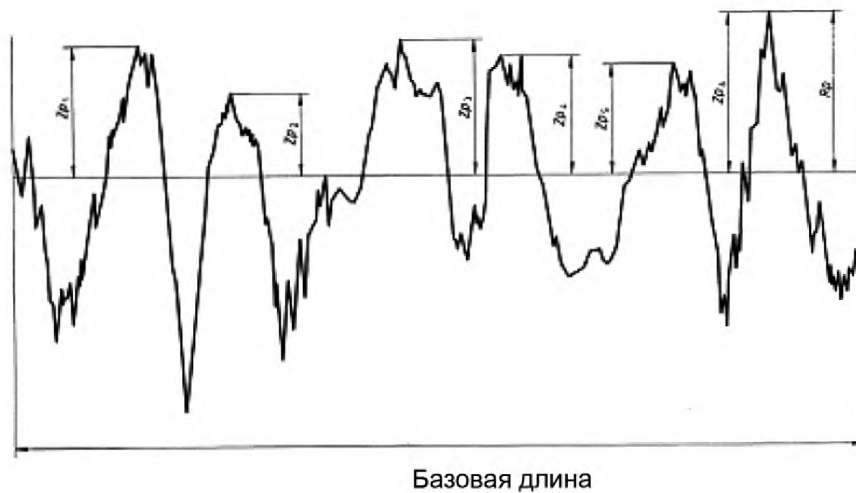
Рисунок 6 — Максимальная высота пика профиля (пример профиля шероховатости)
