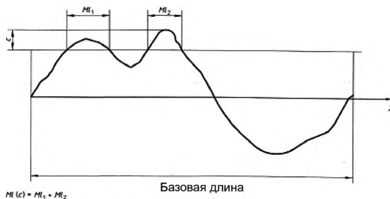
Рисунок 5 — Длина материала
