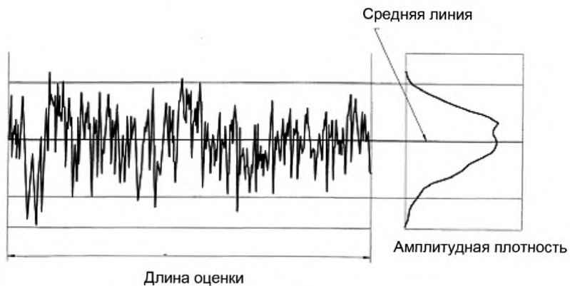
Рисунок 13 — Кривая распределения амплитуд высоты профиля
