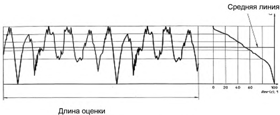
Рисунок 11 — Кривая коэффициента смятия
