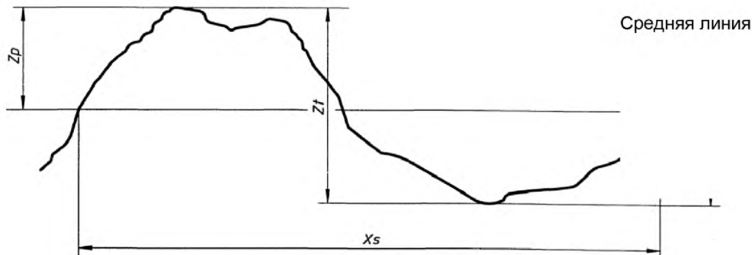
Рисунок 3 — Элемент профиля
