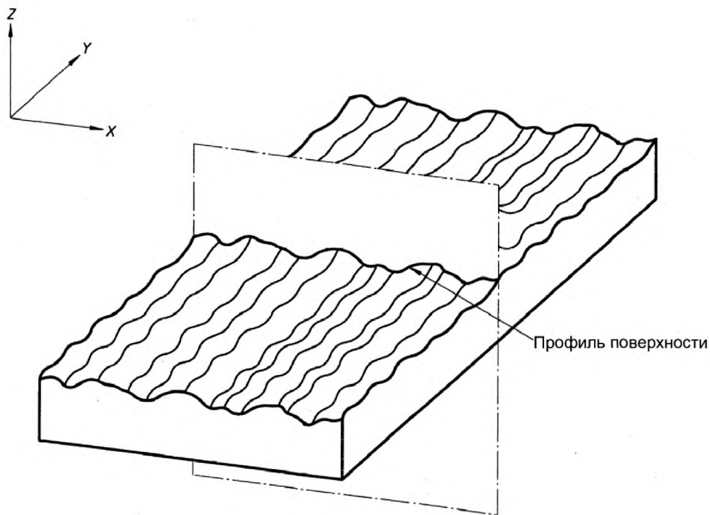
Рисунок 2 — Профиль поверхности
