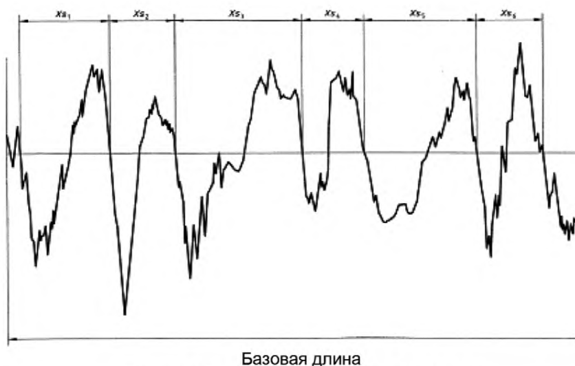
Рисунок 10 — Ширина элементов профиля
