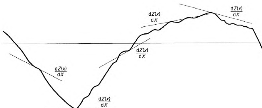
Рисунок 4 — Местный угол наклона
