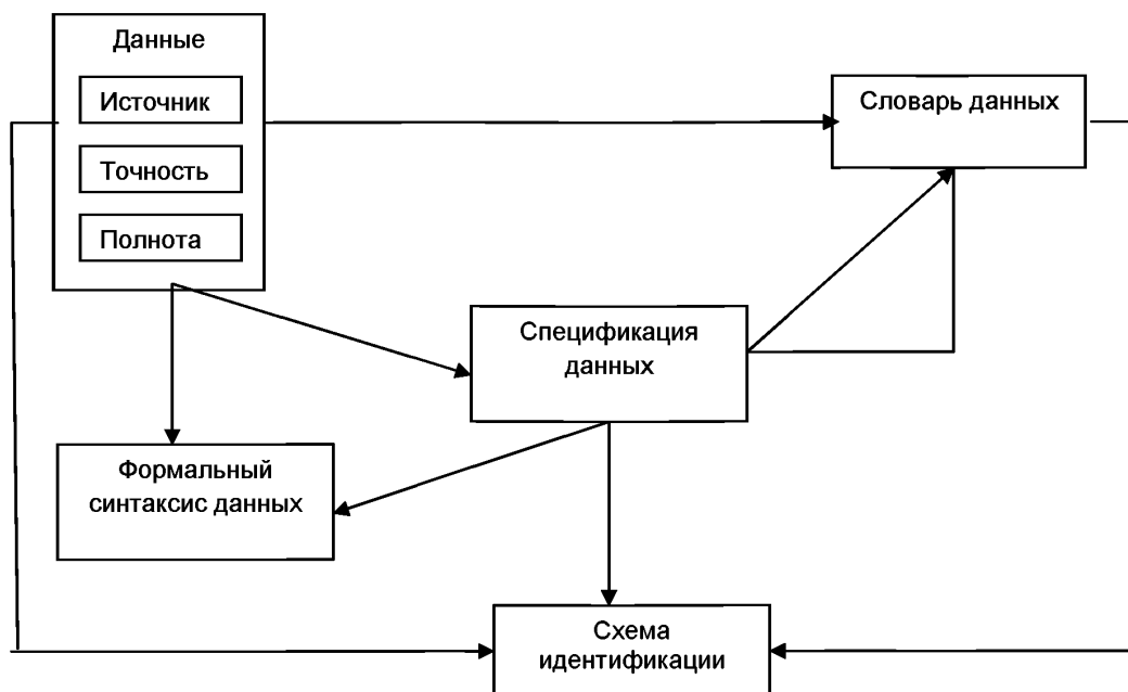
Рисунок 1 – Структура данных
