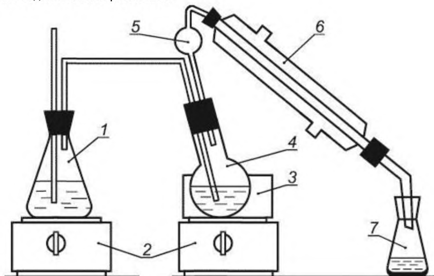
1 – парогенератор, 2 – колбонагреватели, 3 – масляная баня, 4 – перегонная колба с продуктом, 5 – каплеуловитель, 6 – холодильник, 7 – приемная колба
