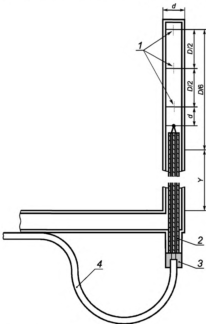
1 — точки отбора проб; 2 — керамическая трубка с двумя каналами; 3 — изолирующий цемент; 4 — провода термопары (хромель — алюминель)
