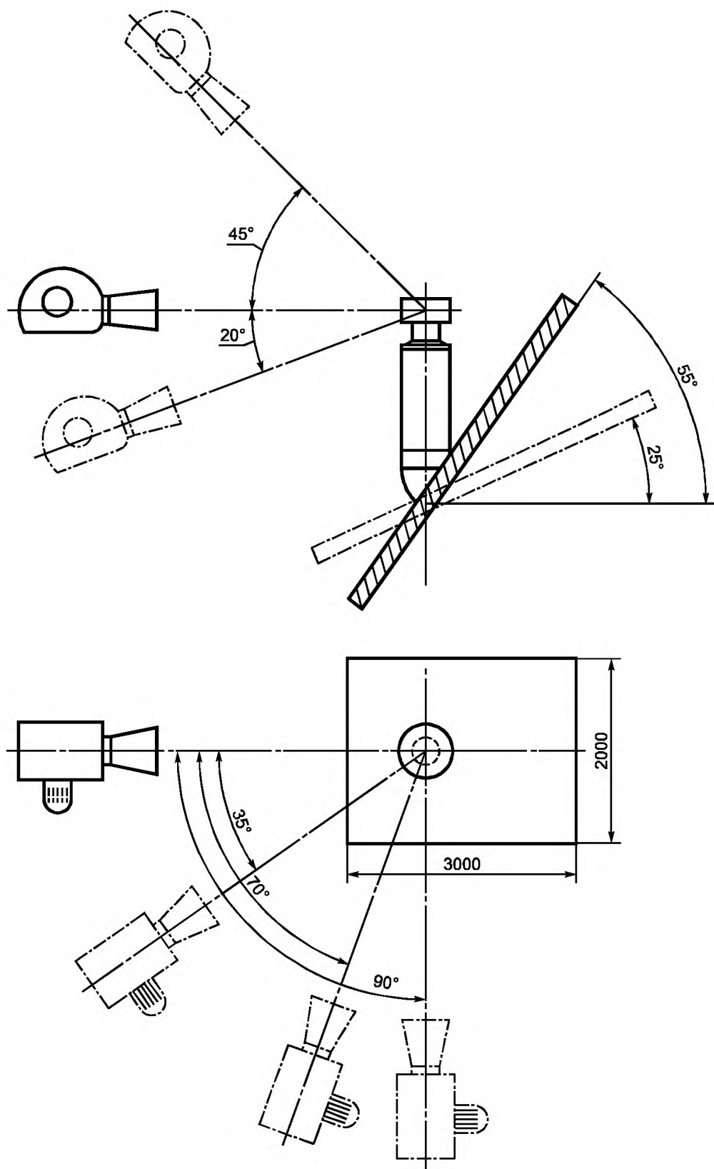
б) испытательный стенд для приборов типа С 3 , оборудованных вертикальным терминалом на наклонной крыше
