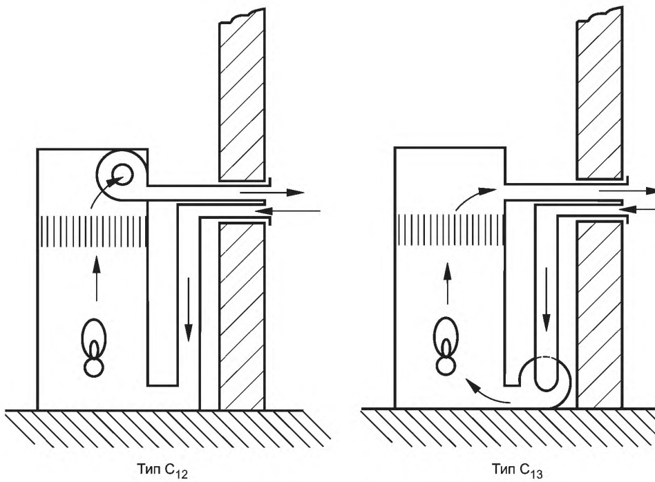
Рисунок В.3 — Схемы приборов типа C 1
