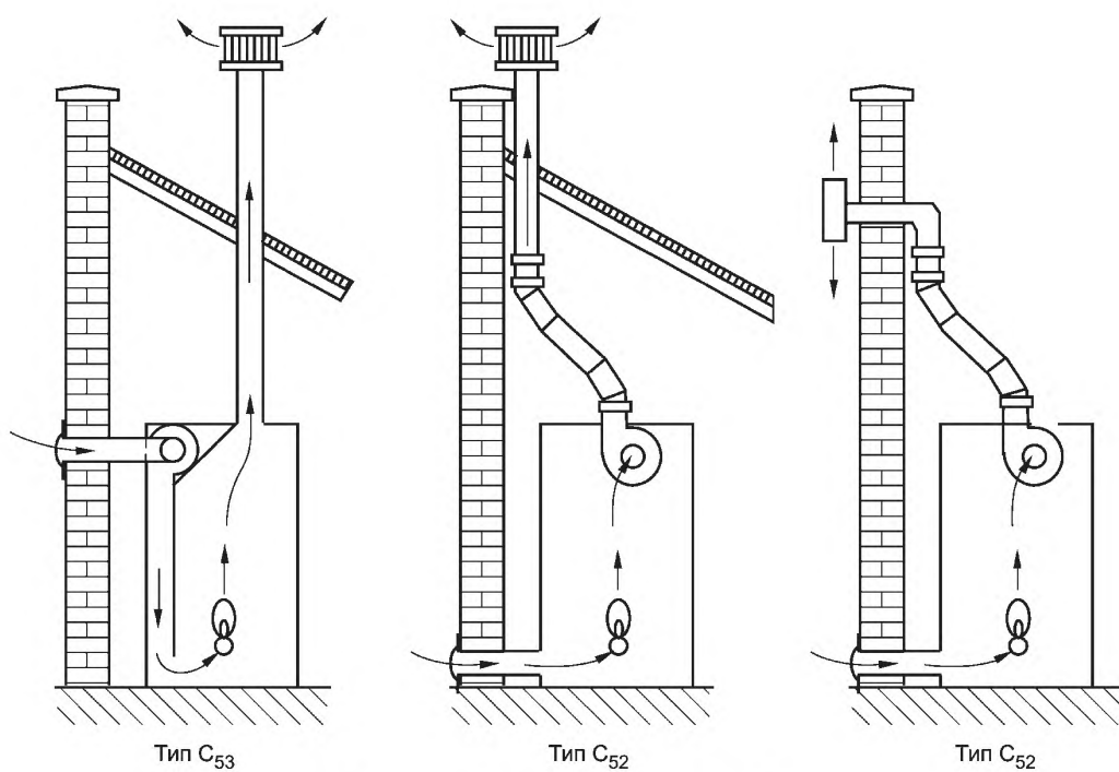
Рисунок В.5 — Схемы приборов типа C 5
