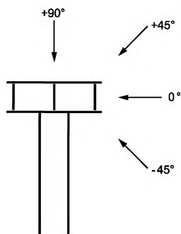
Рисунок С.3 — Скорости ветра
