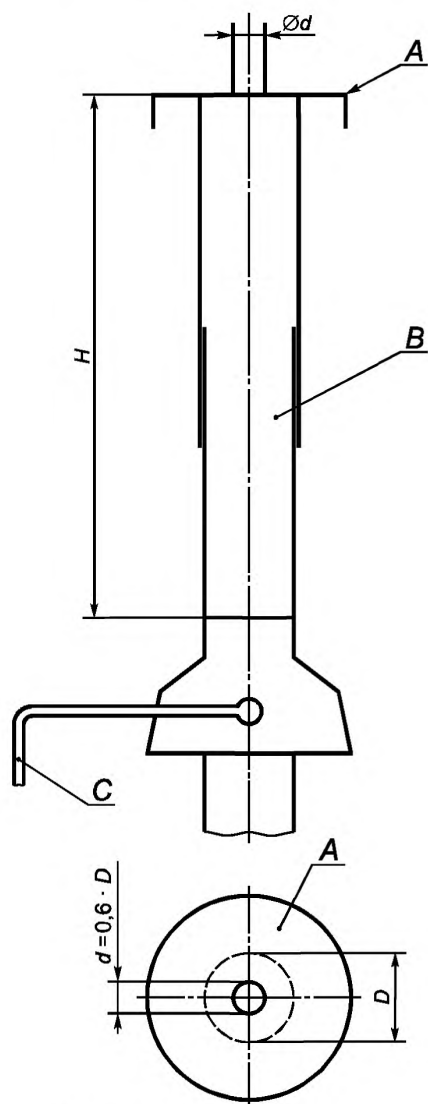
А — пластина; В — телескопический испытательный дымоход; С — датчик тяги; Н — высота испытательного дымохода
