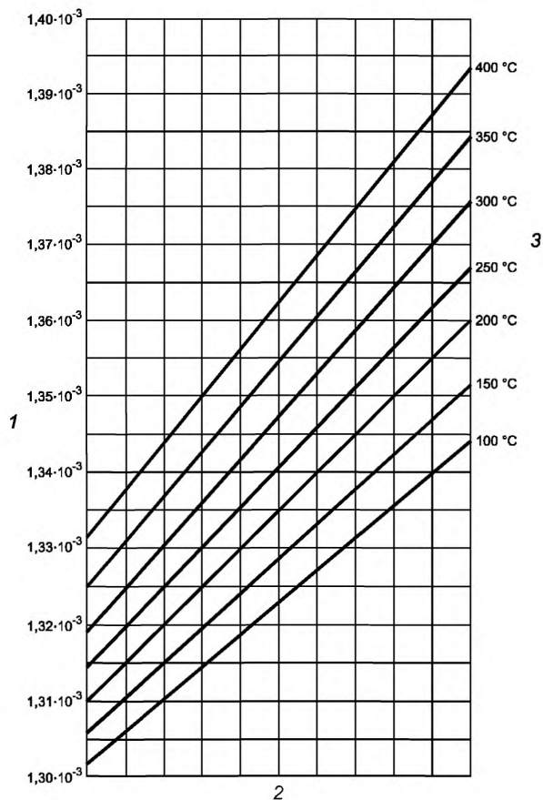
Рисунок 12 — Средняя удельная теплоемкость продуктов сгорания
