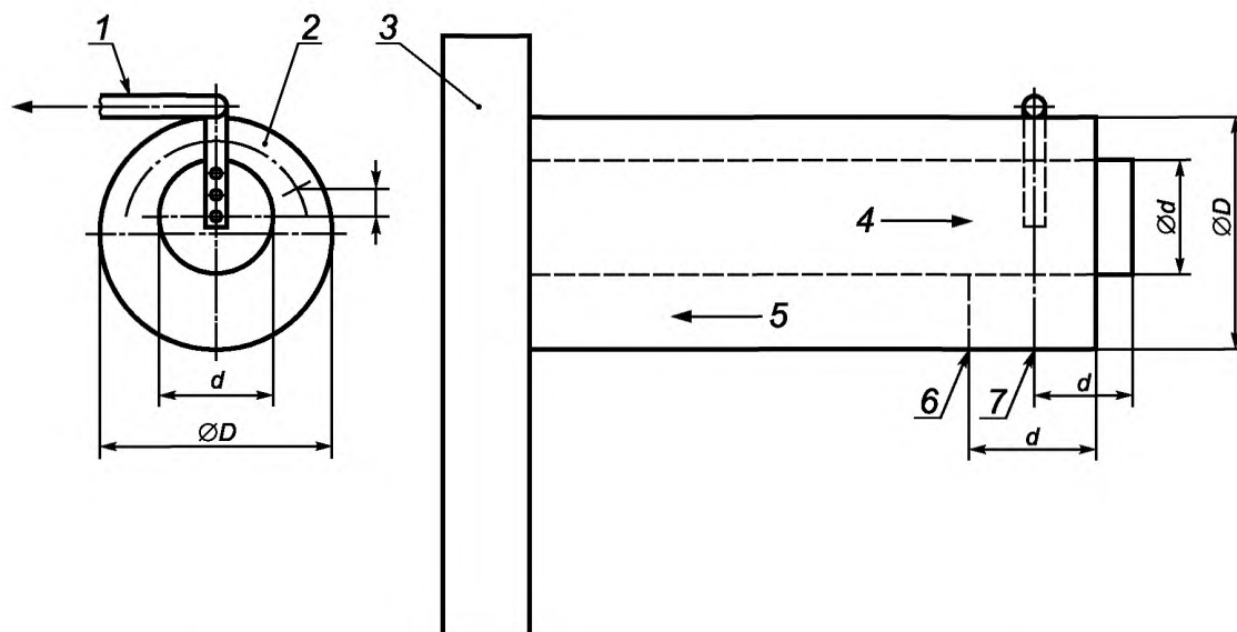
1 — пробоотборник; 2 — воздух для горения; 3 — камера сгорания; 4 — продукты сгорания; 5 — воздух; 6 — сечение для измерения температуры воздуха для горения; 7 — сечение для измерения температуры продуктов сгорания и дымохода
