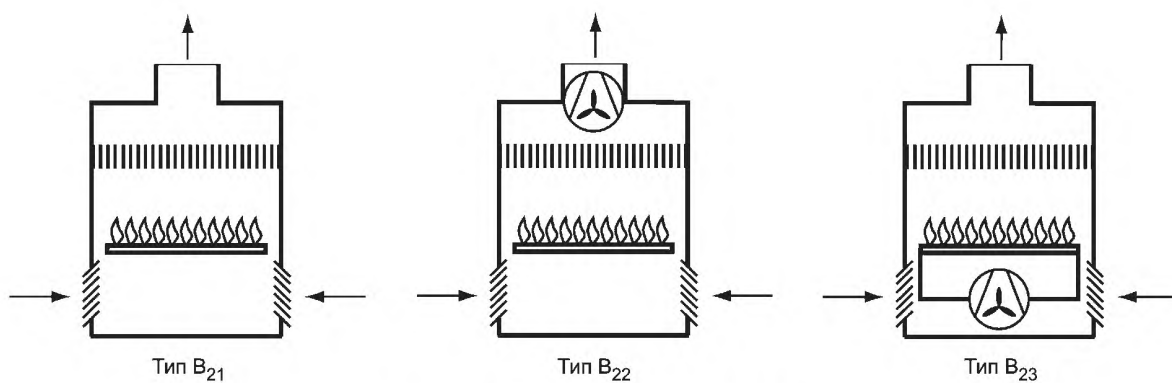
Рисунок В.2 — Схемы приборов типа В 2
