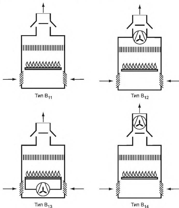
Рисунок В.1 — Схемы приборов типа В 1
