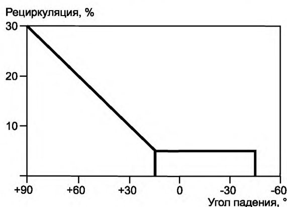
Рисунок С.1 — Максимальная допустимая рециркуляция продуктов сгорания
