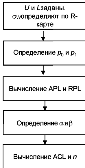
Рисунок 3 – Блок-схема процедуры вычислений (определение элементов APL и RPL)
