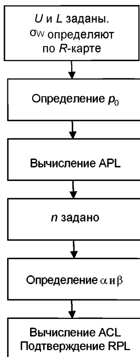
Рисунок 4 – Блок-схема процедуры вычисления (определение элементов APL, \alpha , \beta и n )
