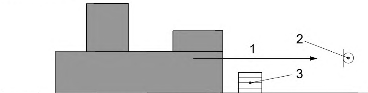
1 – доминирующее направление излучения испытуемого источника; 2 – место установки микрофона; 3 – предпочтительное место расположения образцового источника шума
