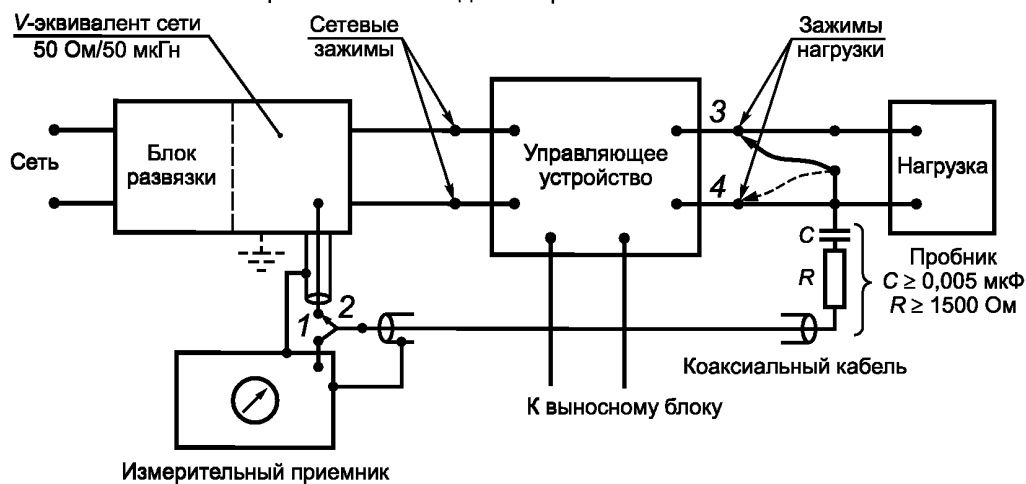
1 — для измерений на сетевых зажимах; 2 — для измерений на зажимах нагрузки; 3 и 4 — последовательные подключения при измерениях на зажимах нагрузки
