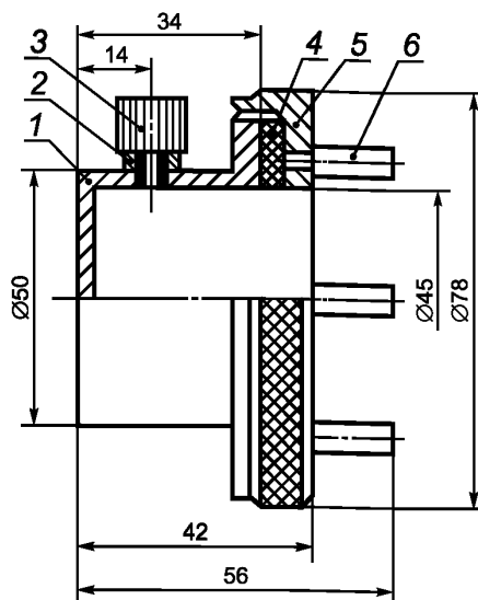
Рисунок 3 — Диффузионная ячейка для испытания гравиметрическим методом
