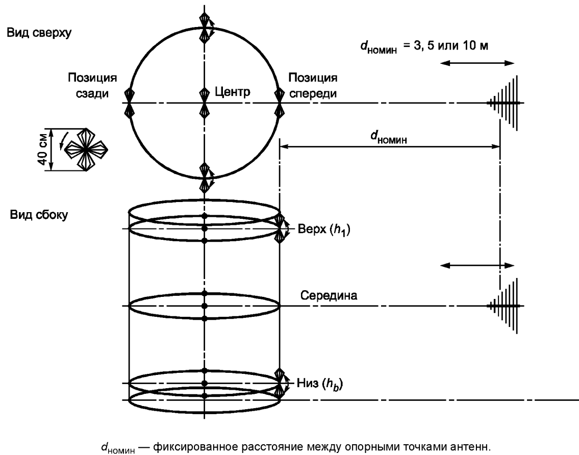
Рисунок 8 — Измерительные позиции антенн при процедуре валидации измерительной площадки
