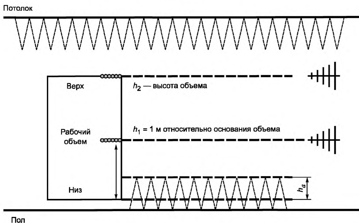
Рисунок 16 — Позиции при измерении KCB_H в горизонтальной плоскости (см. 8.2.2.2.1)
