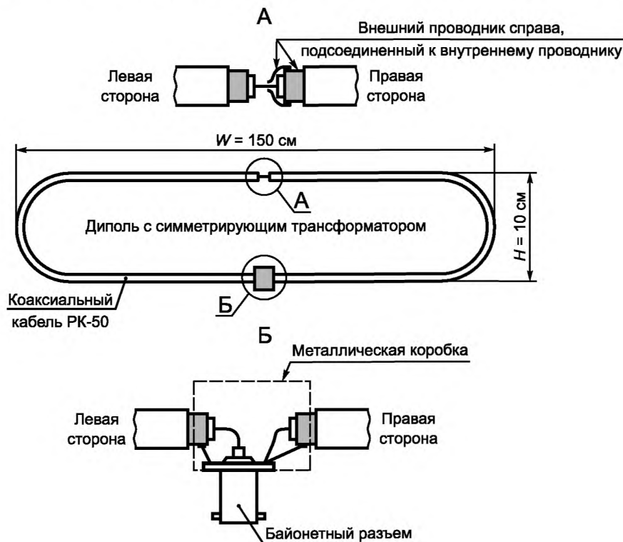
Рисунок В.9 — Конструкция диполя с симметрирующим трансформатором
