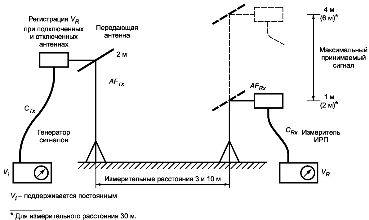
Рисунок 4 — Расположение оборудования для измерения затухания площадки при горизонтальной поляризации (см. 5.6 и приложение Е)
