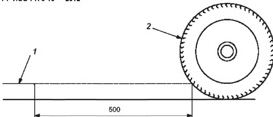
Рисунок 2 — Измерение разбега
