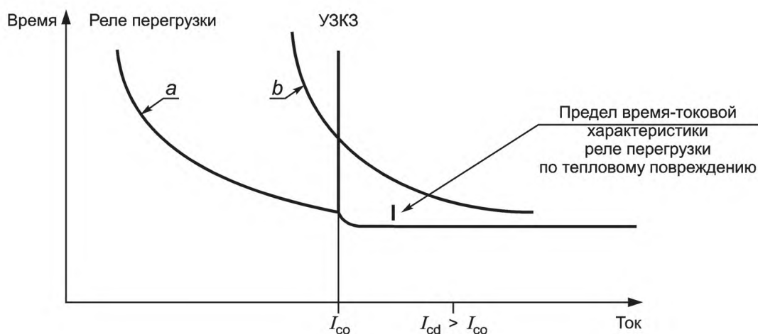
Рисунок В.1b — Координация с автоматическим выключателем
