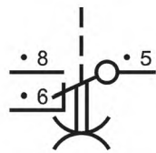
Переключающий контакт с замедлением в обоих направлениях
