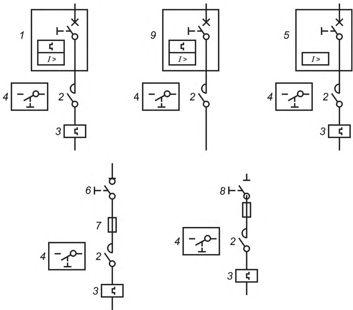
1 — автоматический выключатель; 2 — контактор; 3 — реле перегрузки; 4 — выключатель цепи управления; 5 — автоматический выключатель с одним только электромагнитным расцепителем; 6 — выключатель-разъединитель; 7 — плавкий предохранитель; 8 — разъединитель с плавким предохранителем; 9 — автоматический выключатель с расцепителем перегрузки, соответствующим настоящему стандарту
