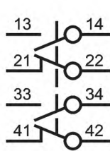
Четыре контактных элемента
