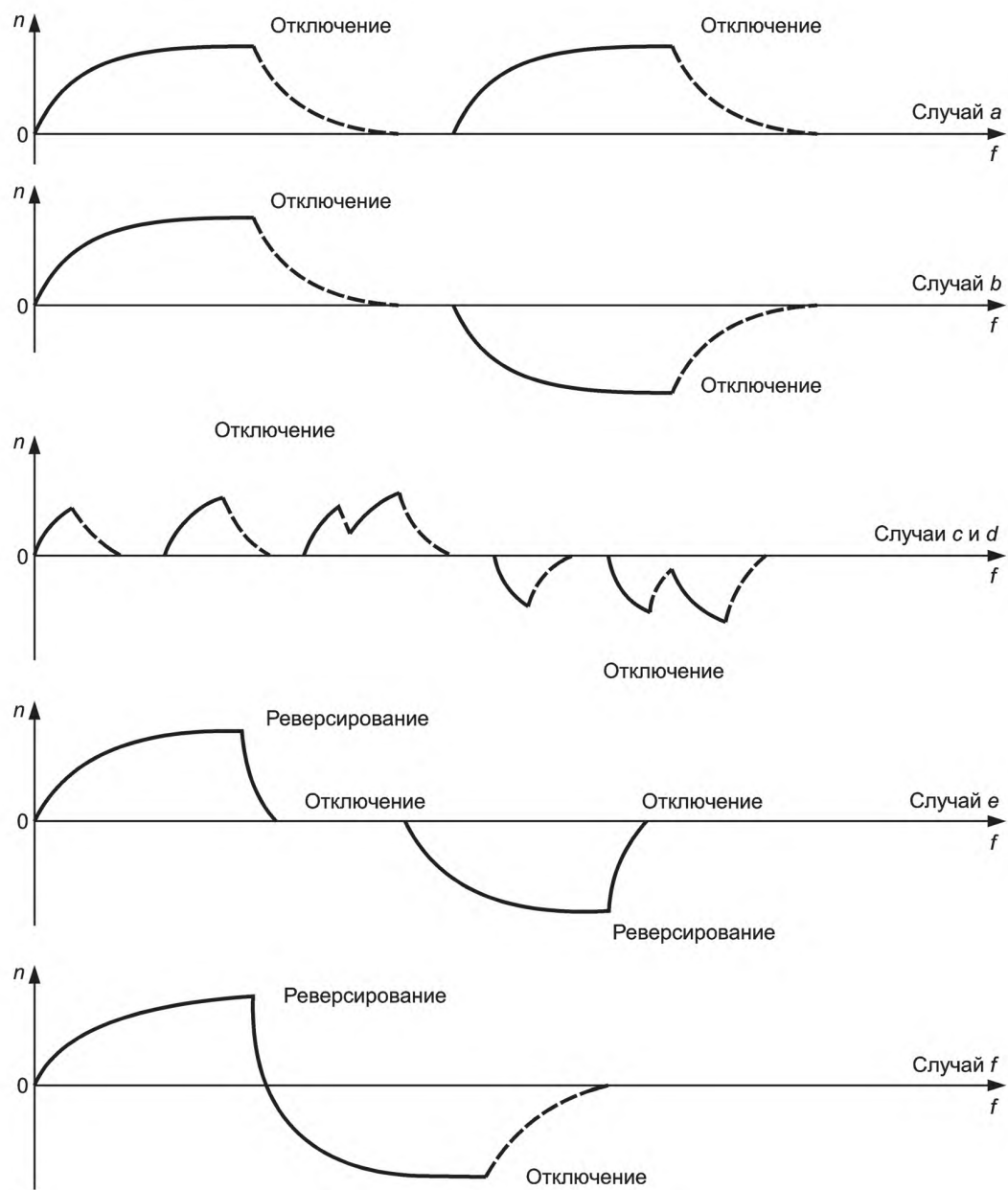
Рисунок 6 — Примеры кривых скорость — время, соответствующие случаям перечислений а)–f) 5.3.5.5 (пунктирные участки кривых обозначают периоды обесточивания двигателя)
