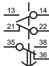
Три контактных элемента
