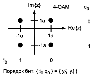
Рисунок 39 — SM 4-QAM отображение с соответствующей битовой комбинацией
