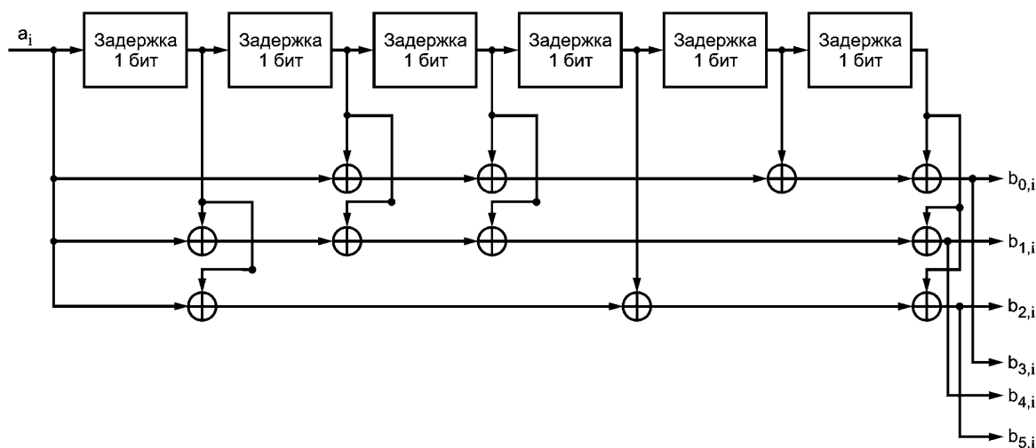
Рисунок 34 — Сверточный кодер
