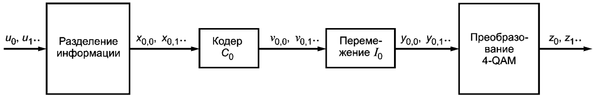
Рисунок 33 — Многоуровневое кодирование с 1 уровнем (SM)
