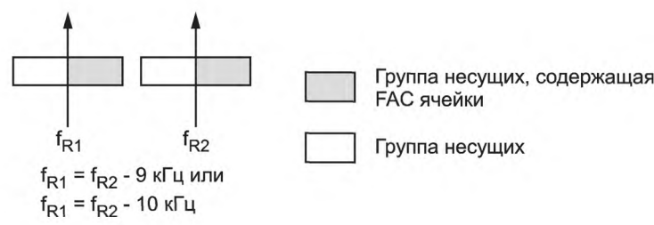
Рисунок М.6 — Пример базового/расширенного DRM сигналов
