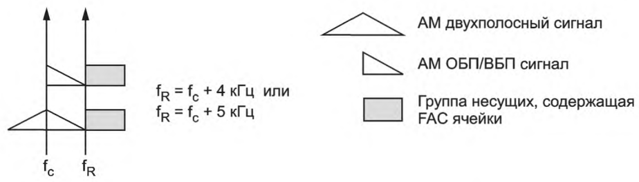
Рисунок М.3 — Пример режимов одновременного вещания для сдвигов на половину канала
