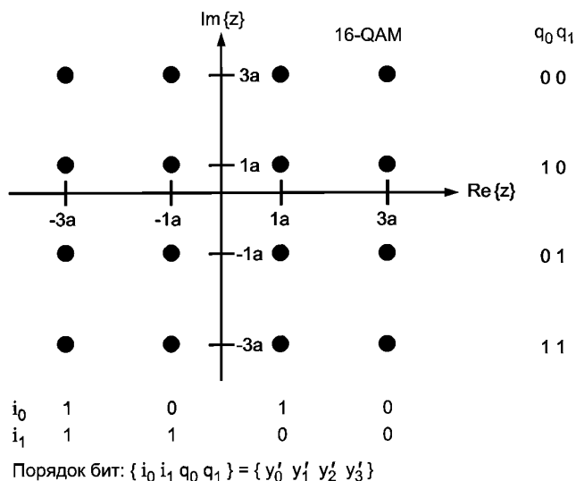
Рисунок 38 — SM 16-QAM отображение с соответствующей битовой комбинацией
