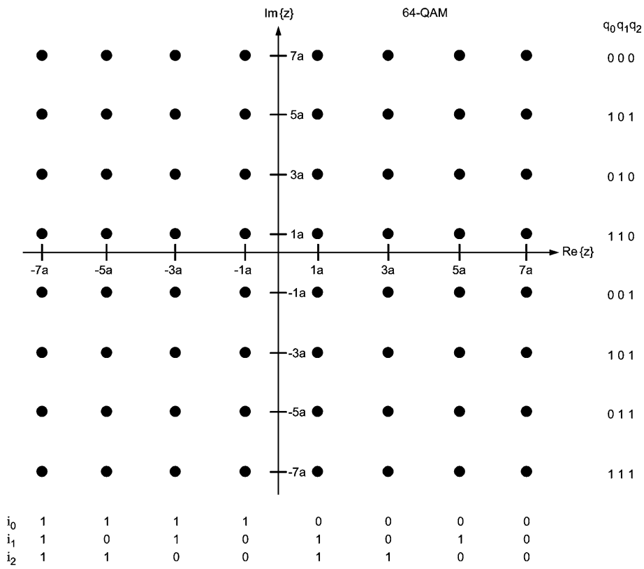
Рисунок 37 — HMTix 64-QAM отображение с соответствующей битовой комбинацией
