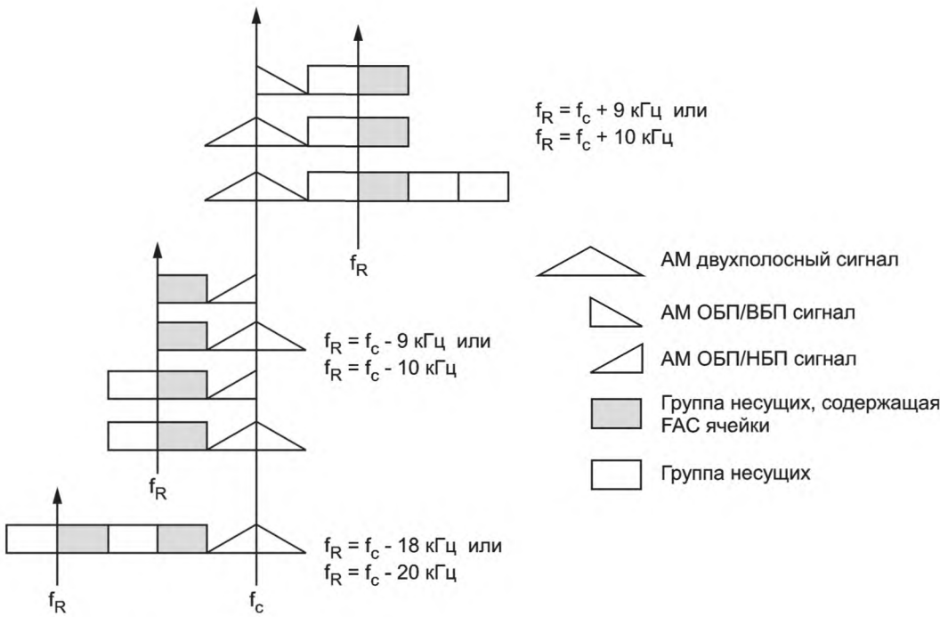
Рисунок М.2 — Пример режимов одновременного вещания для сдвигов на целый канал
