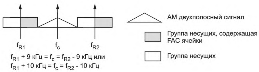
Рисунок М.4 — Пример режимов одновременного вещания с двумя DRM каналами
