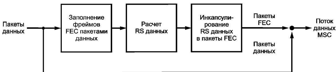
Рисунок 21 — Блок-схема внешнего кодера и внешнего перемежителя
