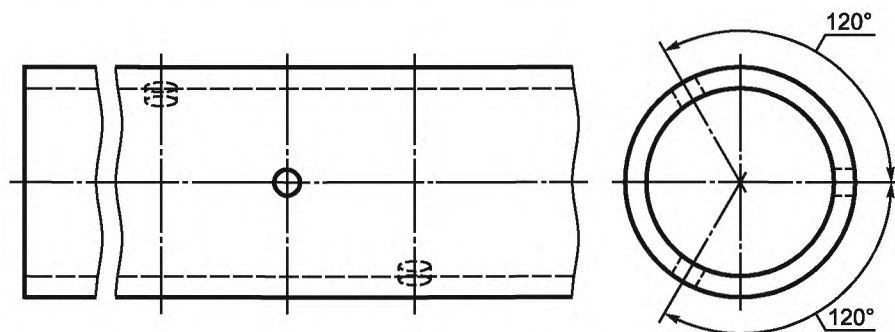
Рисунок Г.1 — Эталонный образец с тремя отверстиями
