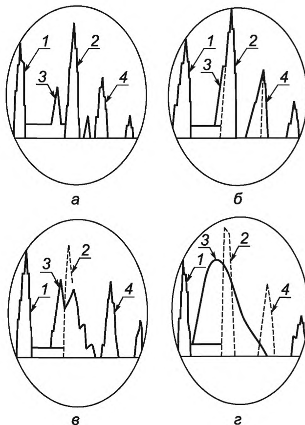
Рисунок В.1 — Вид эхо-сигналов на экране дефектоскопа
