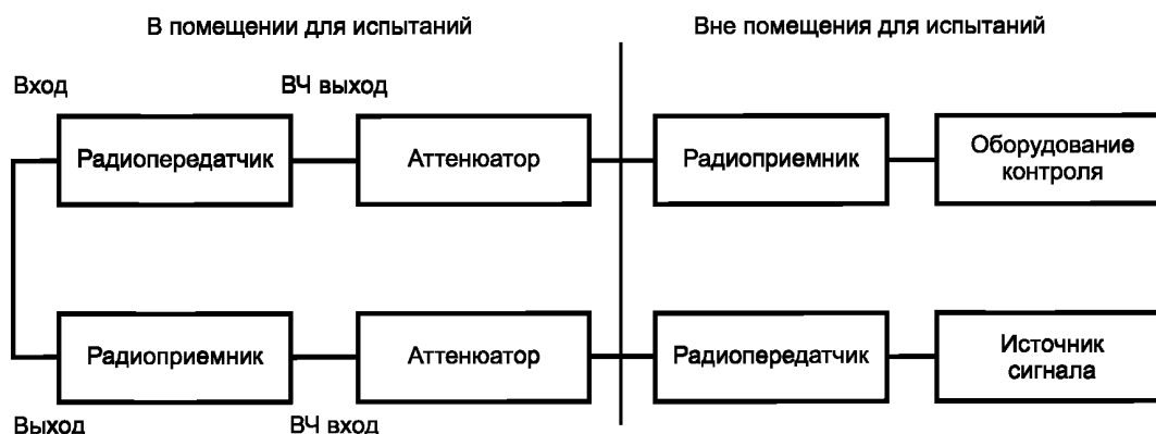
Рисунок 5 — Схема соединений испытываемого приемопередатчика и вспомогательного оборудования при проведении испытаний на помехоустойчивость
