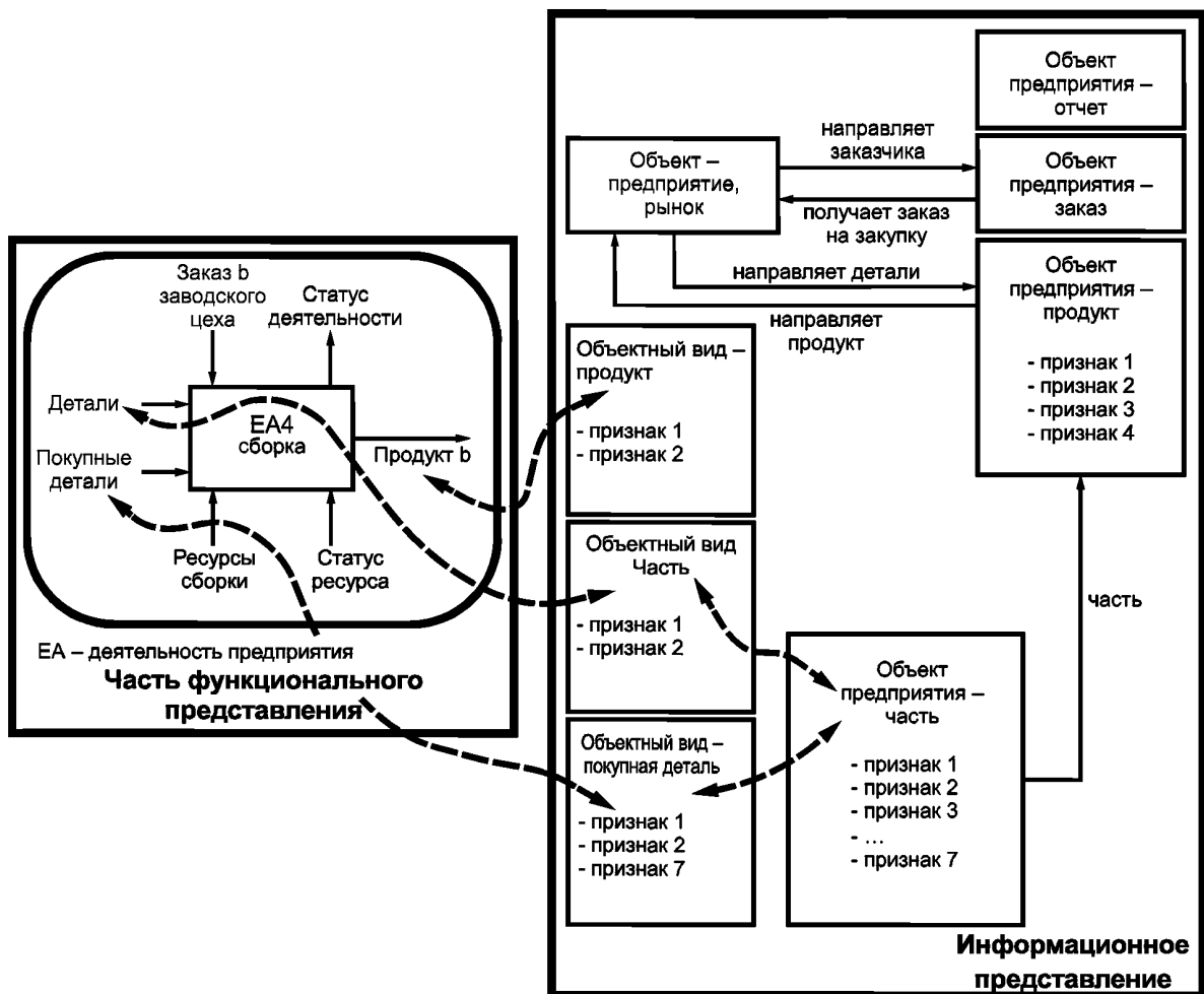
Рисунок В.4 — Информационное представление для обработки заказа
