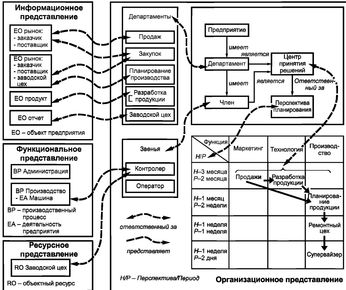
Рисунок В.6 — Организационное представление для обработки заказа
