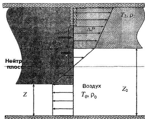
Рис. Пб.1. Массопотоки через проем
