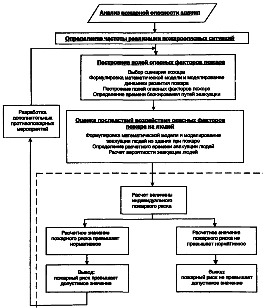
Рис. 1. Порядок проведения расчета индивидуального пожарного риска
