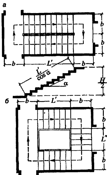
Рис. П5.1. Расчетная длина пути по лестнице:
