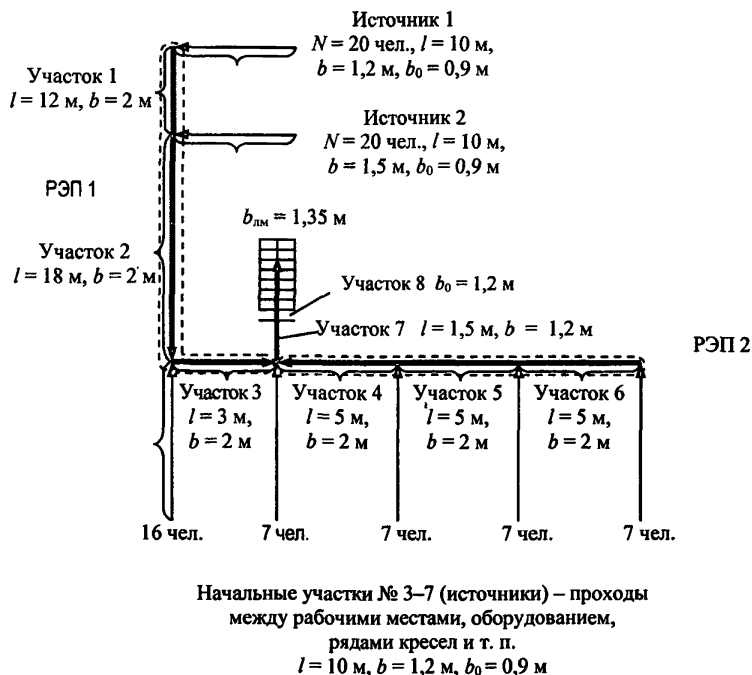
Рис. П5.2. Пример составления расчетной схемы эвакуации людей по части этажа до входа в лестничную клетку:
