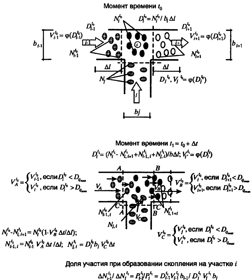
Рис. П4.1. Изменения состояния потока в последовательные моменты времени
