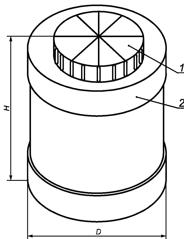
1 — крышка; 2 — корпус
