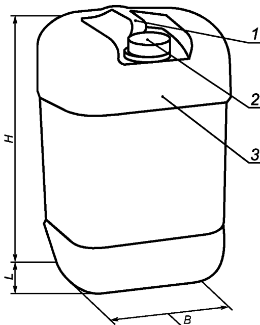
1 — ручка, прикрепленная к корпусу; 2 — крышка; 3 — корпус
