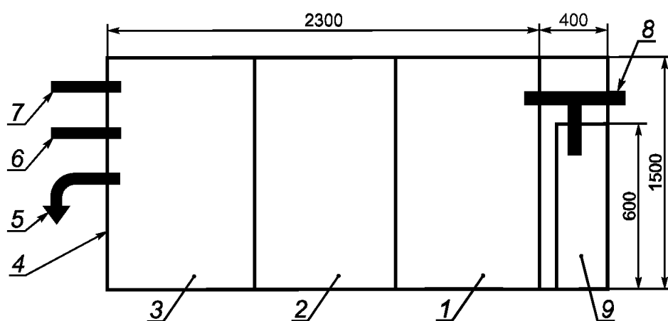
Рисунок 3 — Схема стенда для испытания тары для опасных грузов на штабелирование
