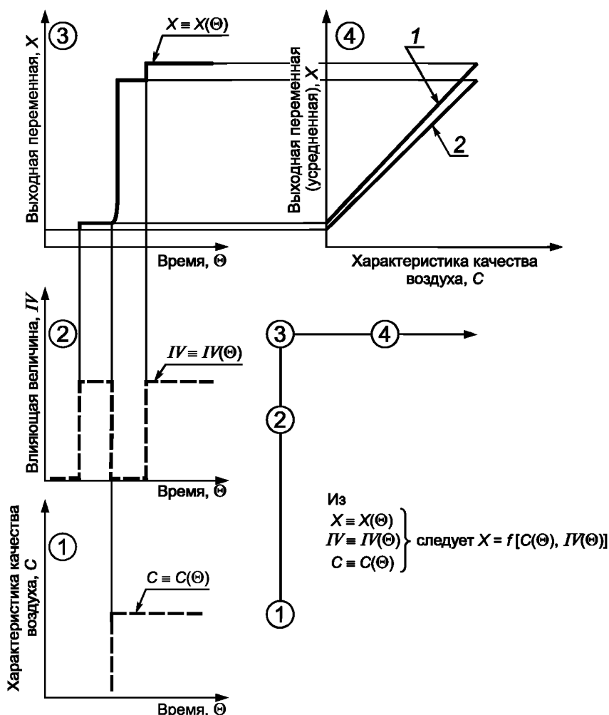
1 — градуировочная характеристика в условиях действия влияющей величины; 2 — градуировочная характеристика в нормальных условиях
