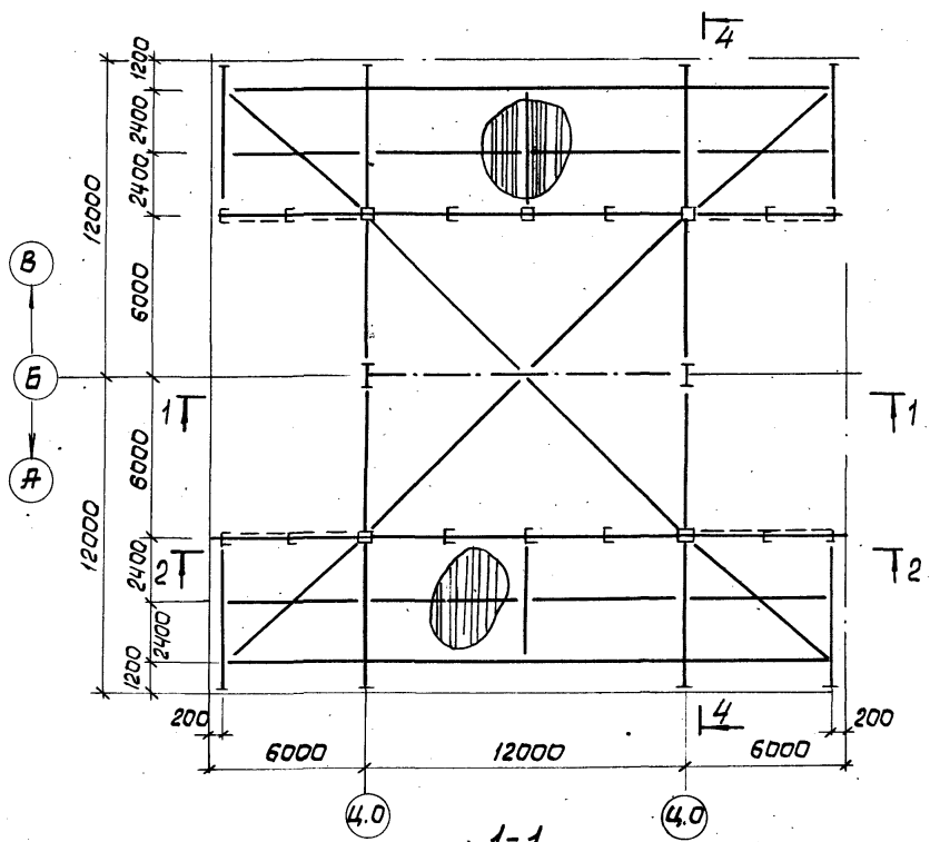
Схема блока БЛ-1
