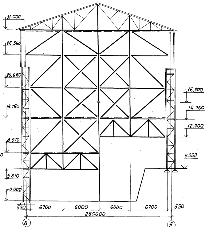
связевой торец
