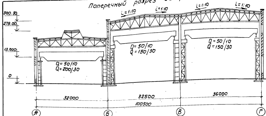
Поперечный разрез цеха после реконструкции.
