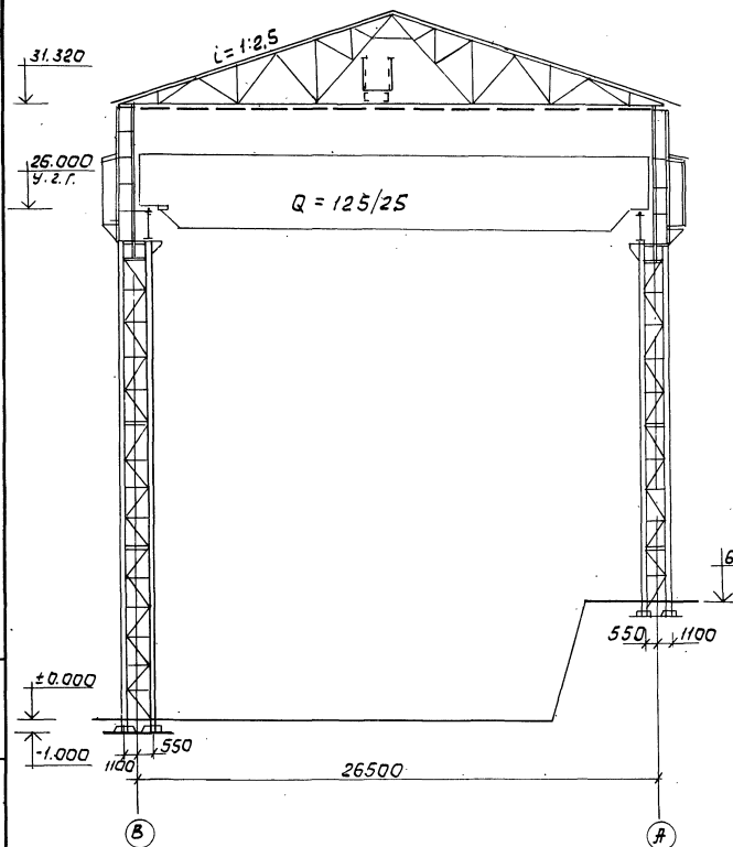
Поперечный разрез
