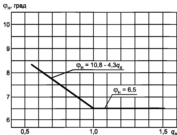
Рисунок 3 — Зависимость угла крена \varphi_n поддресоренных масс АТС от коэффициента поперечной устойчивости q_s
