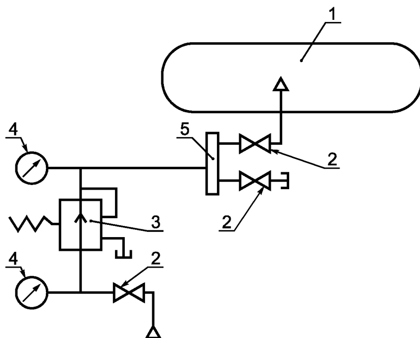
Рисунок Б.2 — Стенд пневматических испытаний
