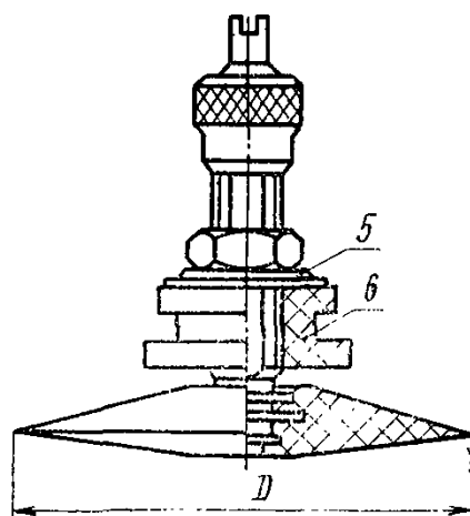
Вентиль РБ
