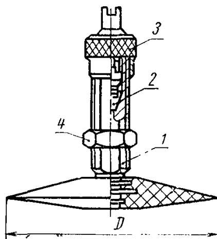
Вентиль РК
