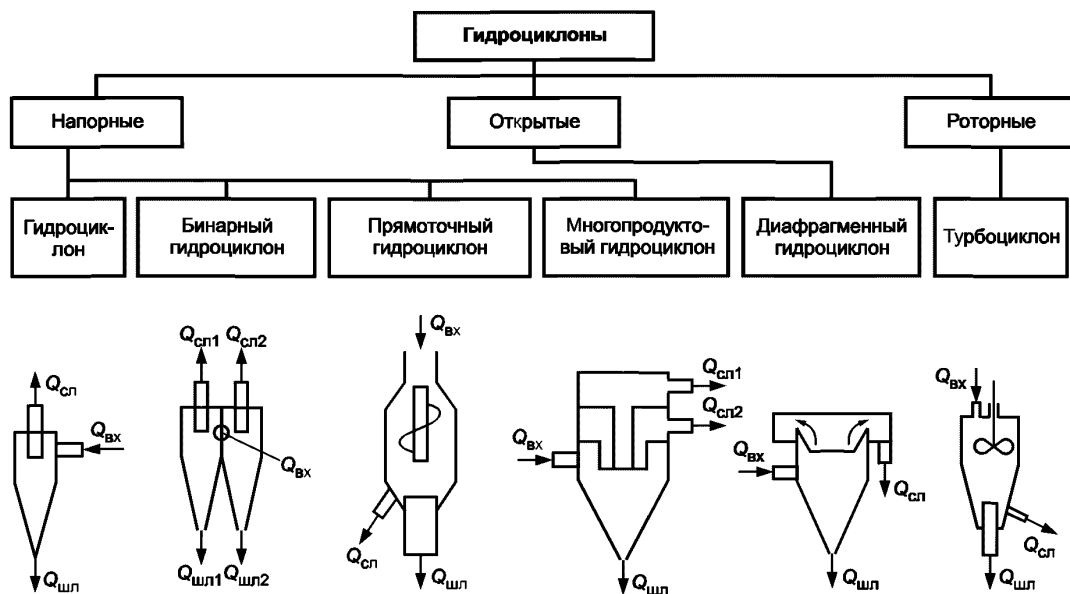
Рисунок 8 — Классификация гидроциклонов
