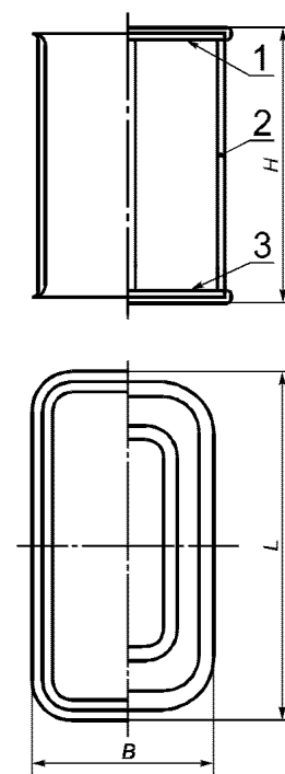
1 — закатное верхнее дно; 2 — корпус; 3 — дно
