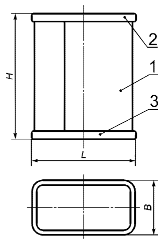
1 — корпус; 2 — съемная крышка; 3 — дно
