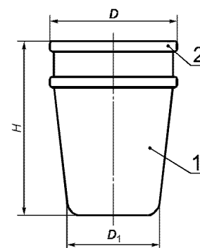
1 — корпус; 2 — закатное верхнее дно
