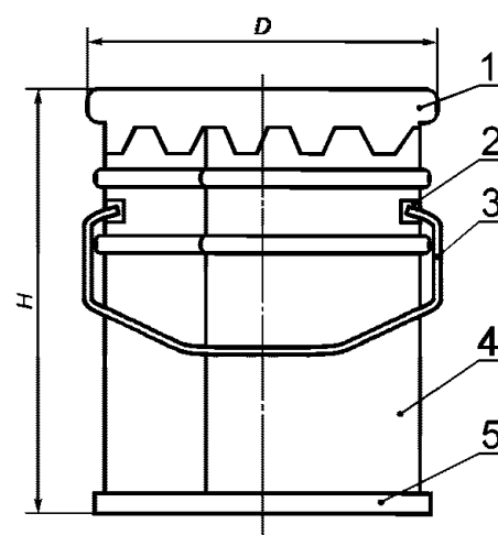
1 — съемная крышка; 2 — накладка для крепления ручки; 3 — ручка; 4 — корпус; 5 — дно
