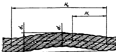
Рис. 2. Волнистость каната
