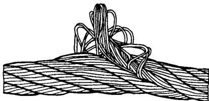
Рис. 4. Выдавливание сердечника
