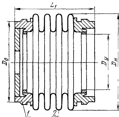
1—присоединительный сильфон патрубок; 2— Черт. 5
