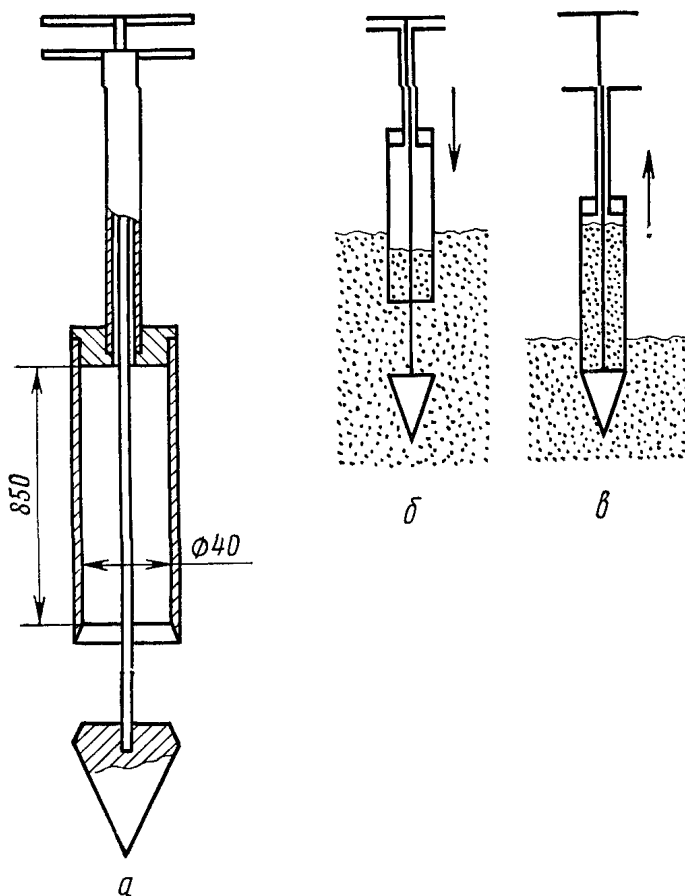
а—схематический чертеж шупа-пробоотборника; б—положение шупа при наборе материала пробы; в—положение шупа при извлечении пробы
