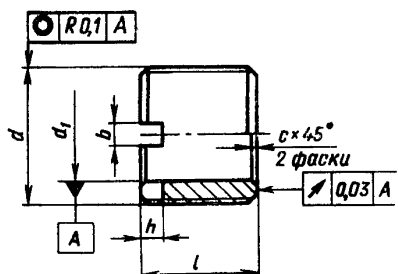
Гайка
