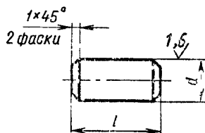
Штифт
