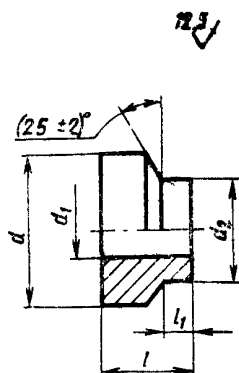
Гайка
