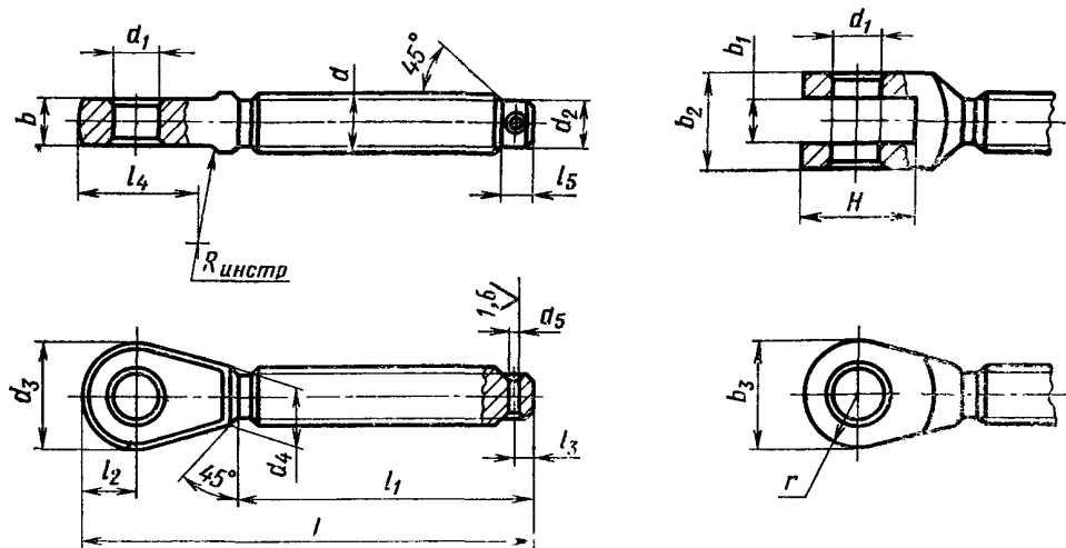
Тяга
