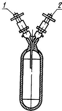
1 2 вентили Черт 1
