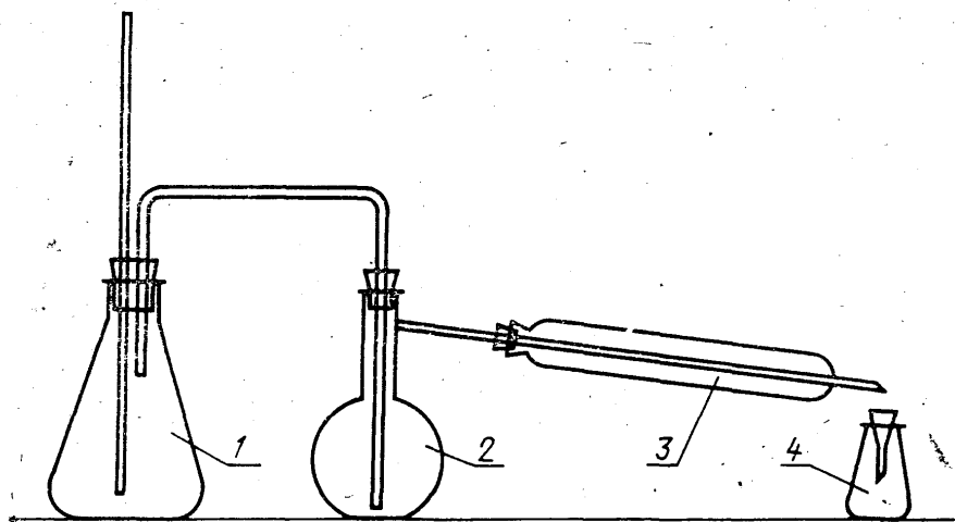
Схема аппарата для отгонки ионола
