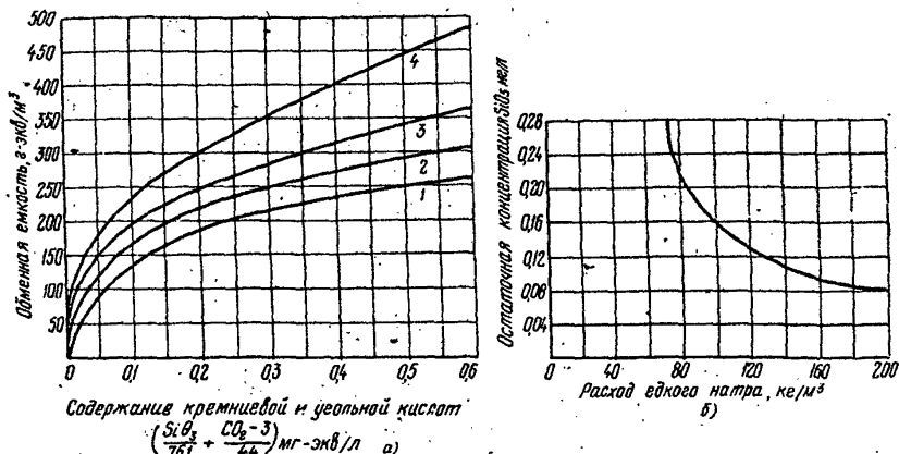
Рис.9. Обменная емкость анионита АВ-17-8 по иону \text{HSiO}_3 для анионитного фильтра второй ступени при обескремнивании воды (при остаточной концентрации \text{SiO}_3 в обессоленной воде не более 0,15 мг/л) и остаточная концентрация \text{SiO}_3 в фильтрате (значения емкости по иону \text{HSiO}_3 даны с учетом концентрации свободной углекислоты в поступающей на фильтр воде 3 мг/л):
