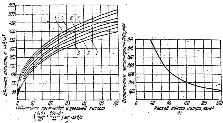
Рис. 11. Обменная емкость анионита АВ-17-8 по иону HSiO_3^- для ступенчато-противоточной технологии обескремнивания воды и остаточная концентрация SiO_2 в фильтрате:
