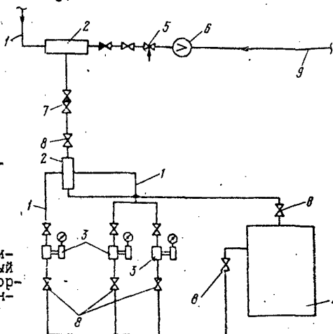
Рис.13. Регенерационный узел подачи серной кислоты:
