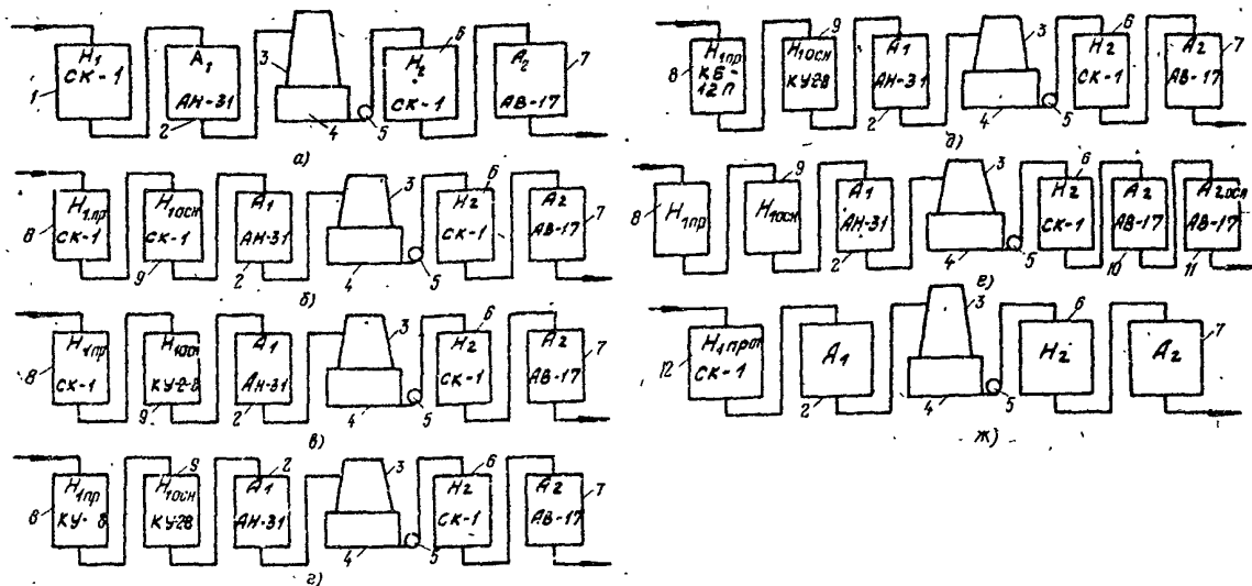
Рис. I. Основные принципиальные схемы обессоливающих установок с блочным включением фильтров:
