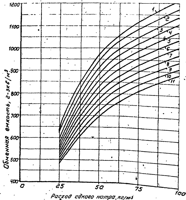
Рис.8. Обменная емкость анионита АН-3И по серной и соляной кислотам при общей концентрации их 0,5-10 мг-экв/л и различных соотношениях кислот (значения для расчета берутся при расходе едкого натра 50 кг на 1 м 3 анионита):
