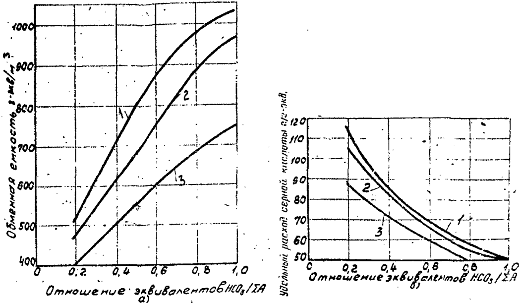
Рис.5. Обменная емкость катионитов и удельный расход серной кислоты на регенерацию пары катионитов КБ-12П и КУ-2-8 при ступенчатой противоточной технологии катионирования (соотношение загруженных (объемов катионитов 1:1):
