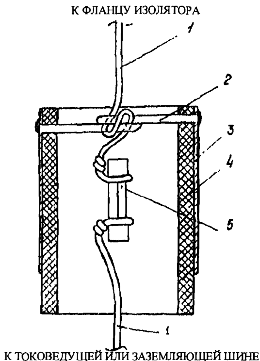
Рис. ПЗ.1. Регистратор перекрытий:
