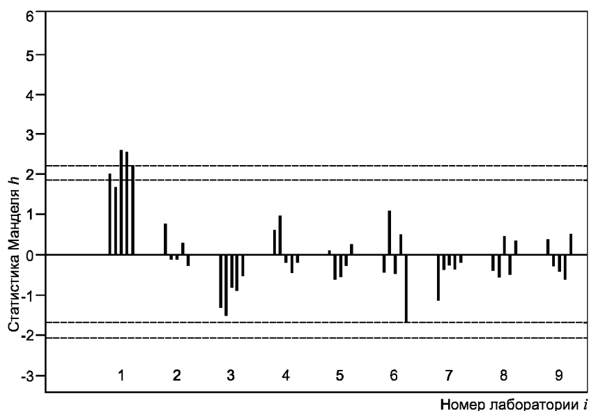
Рисунок В.7 — Титрование крезотого масла. Значения статистики межлабораторной совместимости Мандела h , сгруппированные по лабораториям
